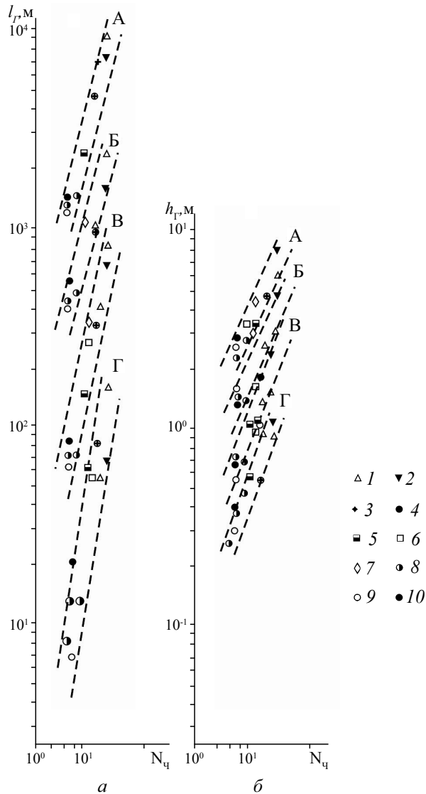
Рис. 4.14. Зависимость длины l_r (а) и высоты h_r (б) град разных типов (А, Б, В, Г) от порядка реки N [Алексеевский, 1987] (1–10 — конкретные реки)
