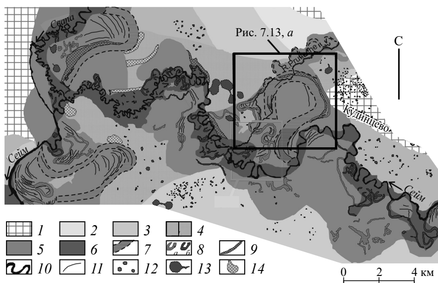
Рис. 7.12. Геоморфологическая карта участка долины р. Сеймы:
