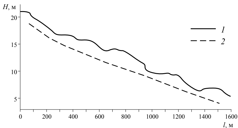
Рис. 3.16. Продольный профиль дна эрозионно-суффозионного понижения в истоках р. Айгурка (бассейн р. Калауса, Ставропольский край):
