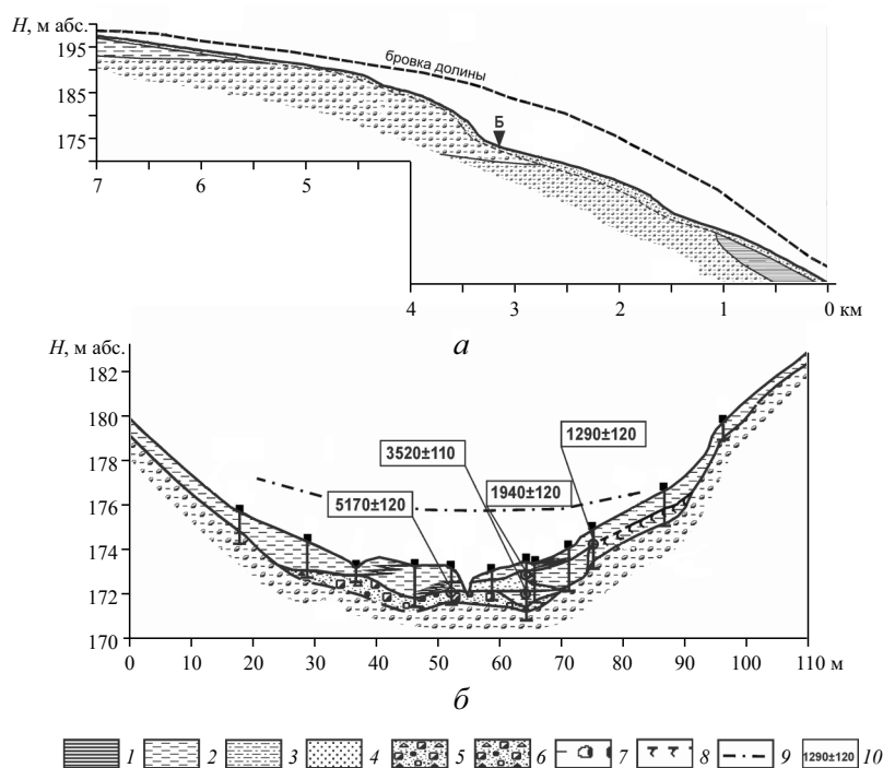
Рис. 7.5. Строение Чолоховской балки (Калужская область, крайняя область московского оледенения) [Беляев и др., 2003, с изменениями]:
