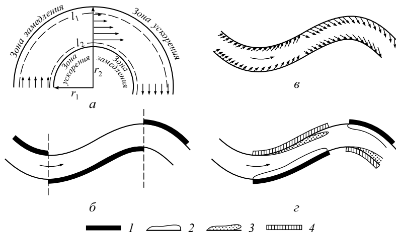
Рис. 4.29. Скоростное поле потока и его воздействие на берега в излучине русла [Маккавеев, 1955]:
