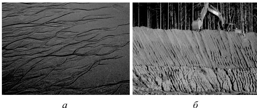
Рис. 1.6. Эрозионные борозды на техногенных склонах: а — струйчатые; б — бороздковые формы размыва поверхности
