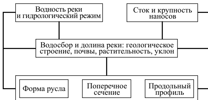
Рис. 4.17. Схема соотношения факторов русловых процессов на участке реки [Craig Fischenich, Hollis Fallen, 2000, с изменениями и дополнениями]
