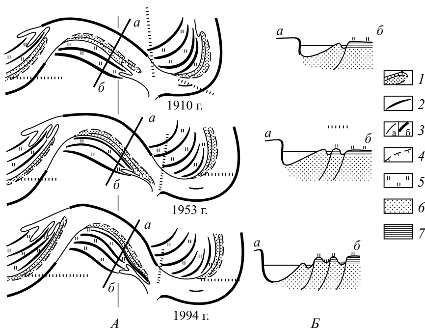
Рис. 4.65. Схема формирования сегментно-гривистой поймы меандрирующей реки (по Р.С. Чалову [1970] с дополнениями А.В. Чернова [1999]):
