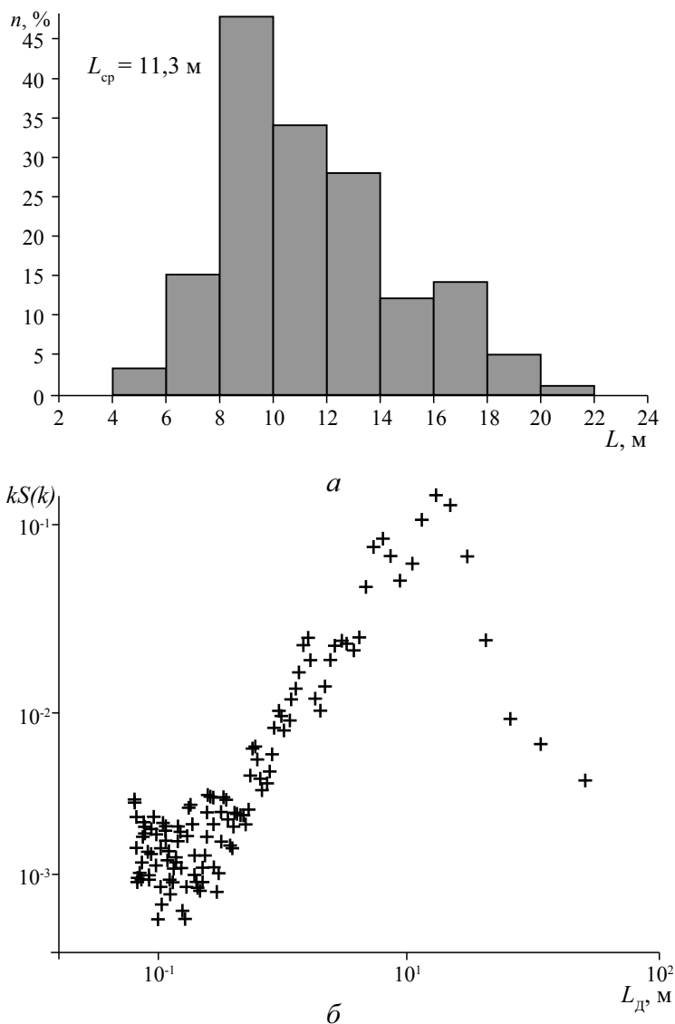
Рис. 4.5. Характеристики длин дюн, полученные методами дискретного (а) и непрерывного (б) анализов (р. Вытегда, перекал Веселый): а — гистограмма длин дюн ( n — число измерений); б — функция спектральной плотности отметок дна kS(k) на единицу длины дюн L_d
