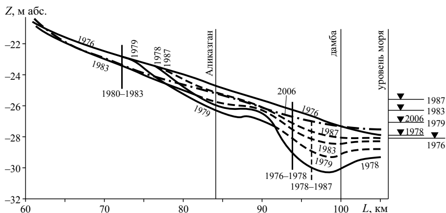
Рис. 5.4. Деформации продольного профиля дна в нижней части устьевое участка Терека [Алексеевский и др., 2007; Гидрология..., 1993].
