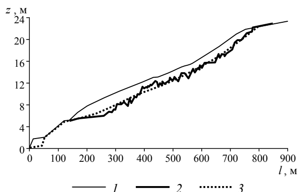
Рис. 3.5. Результаты расчета динамики оврага 9 (Бованенковское месторождение, полуостров Ямал) с помощью динамической модели:
