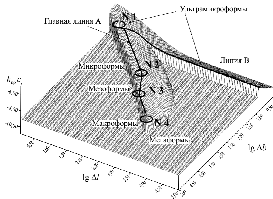
Рис. 4.1. Двумерный спектр волн возмущений дна руслового потока и главные типы этих возмущений (линиями показаны ось двумерных ультрамикроформ и осевая линия максимума спектра; овалами — перегибы осевой линии N_1, N_2, N_3, N_4 и границы между типами возмущений; \Delta l — длины волн возмущений в продольном, \Delta b — в поперечном направлениях; k_{np} c_i — скорости роста амплитуды волн возмущений на единицу длины волн)
