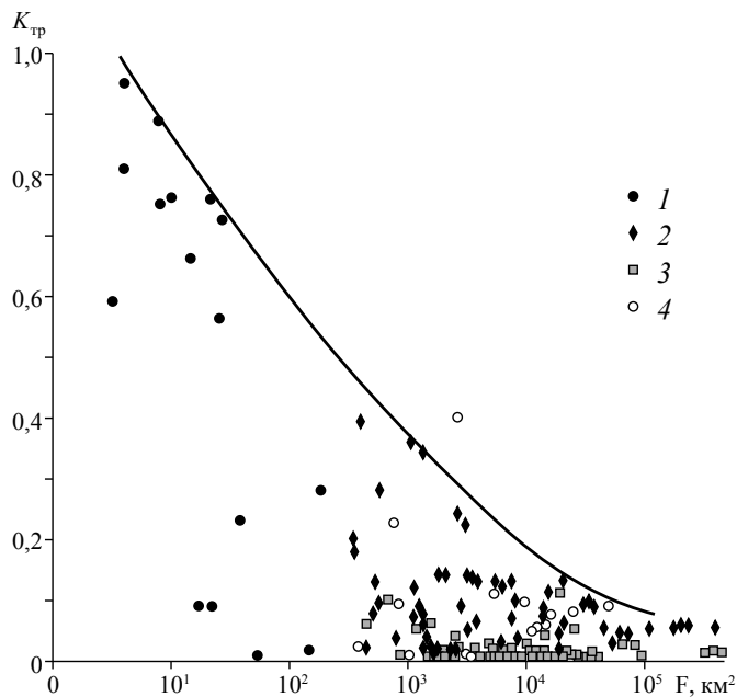
Рис. 1.25. Зависимость коэффициента трансформации стока наносов K_{тр} от площади водосбора реки F , км 2 :
