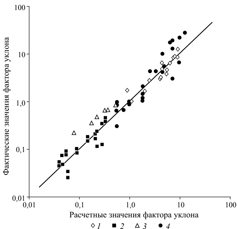
Рис. 2.15. Сопоставление расчетных и фактических значений фактора уклона (по данным: 1 — [Zhongshan, Xiuynq, 1988]; 2 — [Murphree, Mutchler, 1981]; 3 — [Singh, Baby et al., 1981]; 4 — [Нгуен Куанг Ми, 1995])
