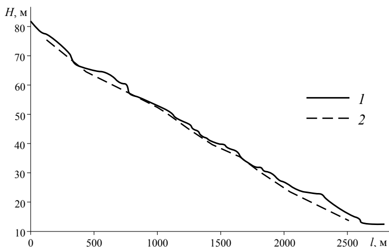
Рис. 3.18. Продольный профиль дна верховьев водосбора Сухой яр (бассейн р. Калауса, Ставропольский край): 1 — современная поверхность дна; 2 — кровля доагрикультурных отложений
