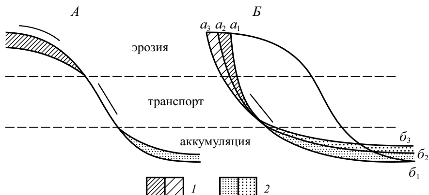
Рис. 1.3. Расположение зон эрозии, транспорта и аккумуляции наносов временными потоками: склоновыми нерусловыми (А), овражными (Б; a_1, b_1, a_2, b_2; a_3, b_3 — последовательные положения продольного профиля оврага); 1 — зона размыва; 2 — зона аккумуляции
