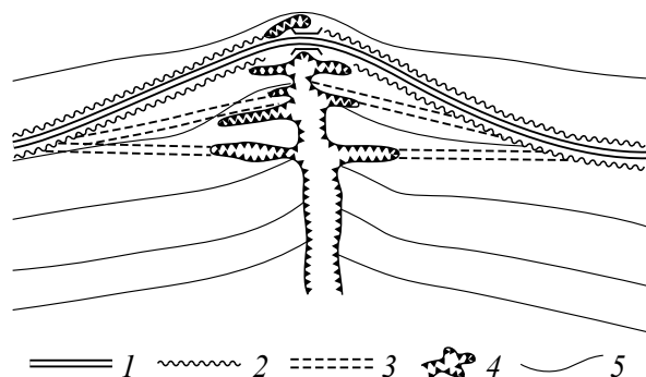
Рис. 3.9. Сеть оврагов, растущих по кюветам при пересечении ложбины шоссевой дорогой: 1 — действующая дорога; 2 — кюветы; 3 — заброшенные дороги; 4 — овраги; 5 — горизонталы [Арманд, 1958]
