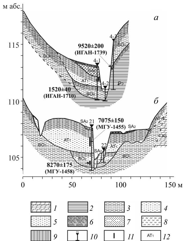
Рис. 7.3. Продукты пирогенной эрозии на водосборе и склонах Берестовой балки (Ростовская область), накопившиеся в ее днище в среднем течении:
