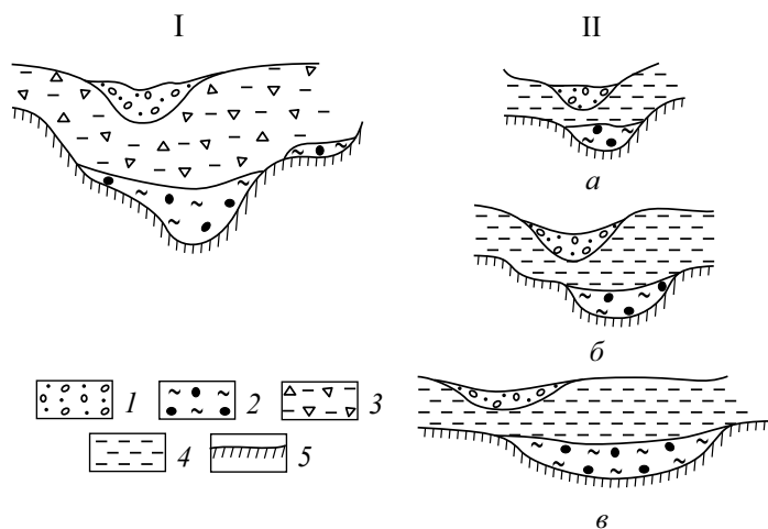
Рис. 7.24. Соотношение ширины днщ современных и погребенных долин в районах: I — Ленском; II — Куларском на участках: а — низкогорного рельефа; б — плоскогорья; в — приморской низменности; 1 — аллювий современных долин; 2 — то же погребенных долин; 3 — флювиогляциальные и гляциальные отложения; 4 — лессовидные суглинки; 5 — коренные склоны
