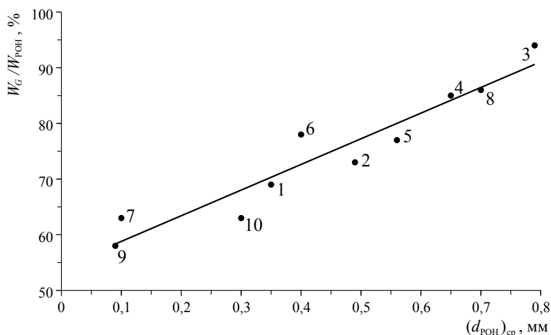
Рис. 4.61. Зависимость доли влекомых наносов в общем стоке руслообразующих наносов от их среднего диаметра (реки: 1 — Днестр; 2 — Чулым; 3 — Ока; 4 — Выгегда; 5 — Белая; 6 — Десна; 7 — Амур; 8 — Неман; 9 — Северский Донец; 10 — Васюган)
