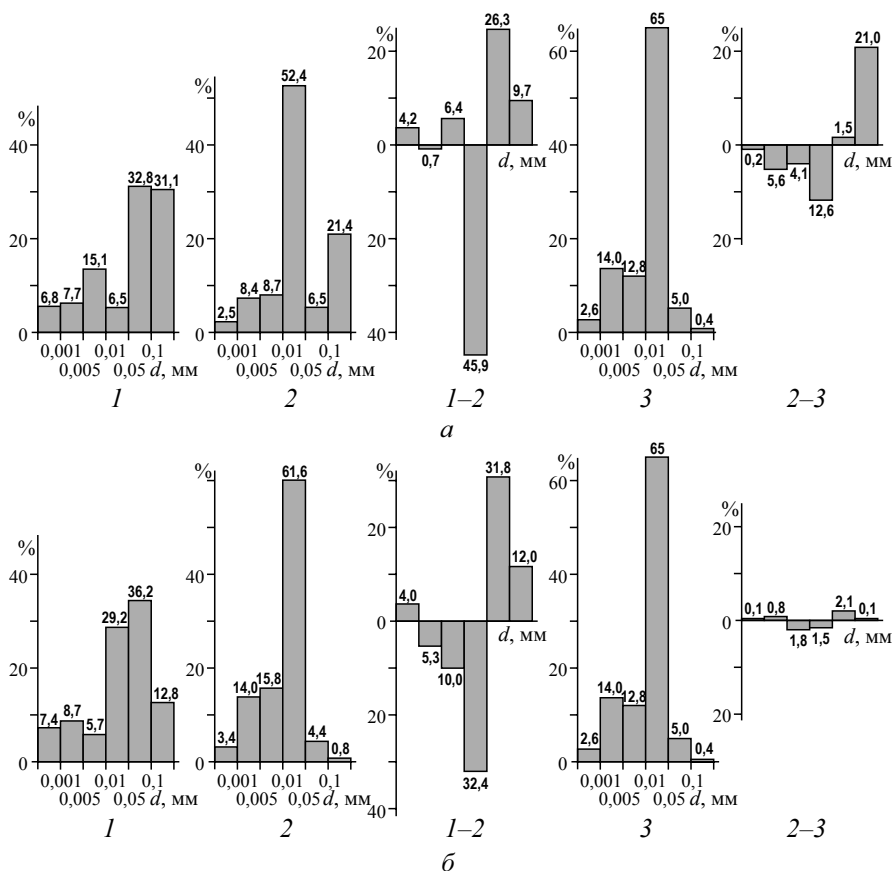
Рис. 6.6. Изменение механического состава наносов в системе склон — русло реки: а — в период прохождения максимальных расходов воды; б — на спаде половодья. Наносы: 1 — речные; 2 — овражные; 3 — склоновые; разница: 1-2 — речных и овражных; 2-3 — склоновых и овражных
