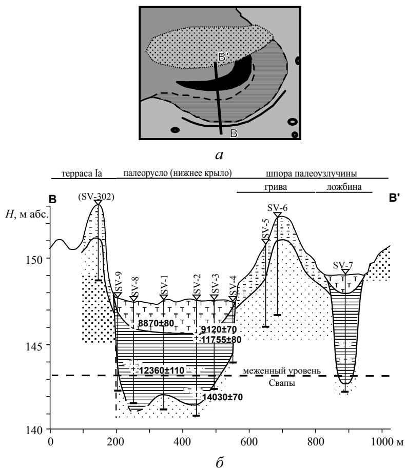
Рис. 7.14. Геологический профиль через палеорусло поздневалдайской макроизлучины р. Свапы у д. Семеновки (условные обозначения — см. на рис. 7.13)
