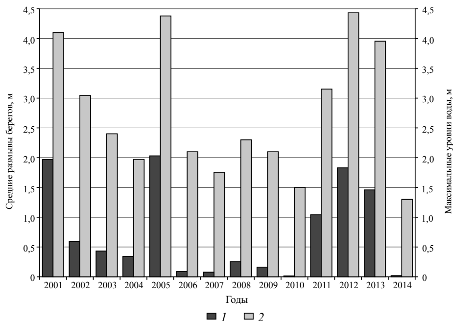
Рис. 4.48. Связь интенсивности размывов вогнутых берегов излучин р. Керженец с высотой половодий (по О.В. Кораблевой и А.В. Чернову [2012], с дополнениями)
