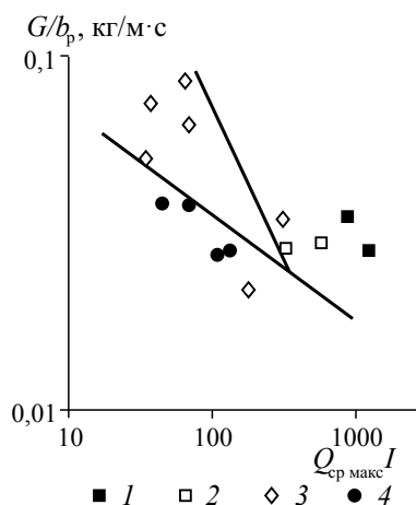
Рис. 4.64. Распределение морфодинамических типов русел на реках бассейна Северной Двины в поле диаграммы мощность потока QI — удельный расход влекомых наносов s_G (разветвления: 1 — сложные, 2 — одиночные; излучины: 3 — петлеобразные, сегментные крутые и прорванные; 4 — прямолинейное неразветвленное русло (по П.Н. Резникову и Р.С. Чалову [2005], с изменениями и дополнениями))
