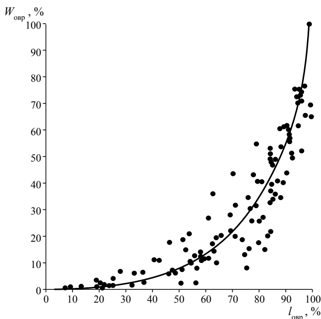
Рис. 3.2. Зависимость между относительным ростом длины оврага I_{\text{овр}} (%) и его объемом W_{\text{овр}} (%)
