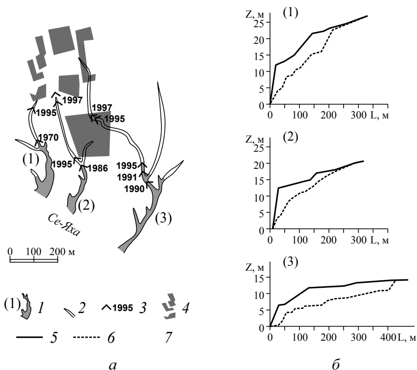
Рис. 1.24. Эволюция планового положения (а) и продольных профилей (б) антропогенных оврагов (1, 2, 3 у поселка комплексного электрохозяйства Бованенковского ГКМ на Ямале): 1 — эрозионный врез антропогенного оврага; 2 — эрозионные ложбины выше оврагов на склоне; 3 — время и положение вершины оврага; 4 — площадки сооружений поселка; 5 — профили склонов; 6, 7 — профили тальвегов оврагов в 1991 и 1995 гг. соответственно
