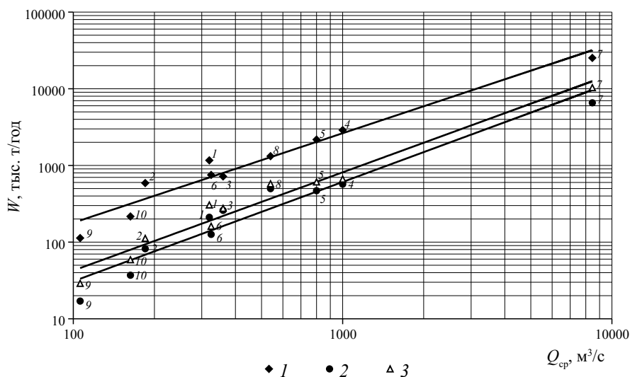
Рис. 4.62. Зависимость стока взвешенных W_R (1), влекомых W_G (2), руслообразующих — влекомых и взвешенных W_{РОН} (3) наносов от среднего многолетнего расхода воды ( Q ) на равнинных реках:
