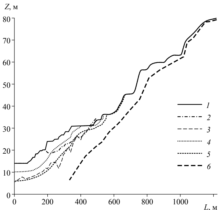
Рис. 3.7. Сопоставление фактического, рассчитанного по динамической модели и прогнозного на 2110 г. продольного профиля оврага Мботма-новый в условиях климата и землепользования
