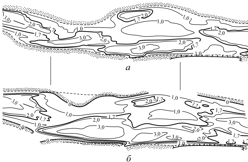
Рис. 4.58. Многолетние изменения отметок дна на смежных Слудских перекатах Северной Двины:
