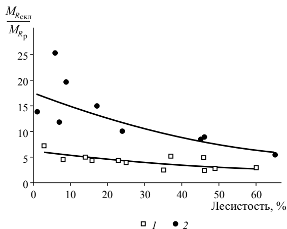
Рис. 6.9. Зависимость доли склонового стока в стоке наносов реки \frac{M_{R_{р}}}{M_{R_{скл}}} от лесистости водосбора для бассейна Оки: 1 — средние и большие реки; 2 — малые реки
