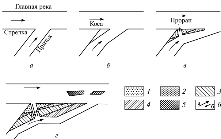
Рис. 4.44. Схема развития пойменно-руслового разветвления в узле слияния рек ( a – з ): 1–5 — последовательные этапы роста стрелки и острова ниже стрелки; б — направления течений в спрямляющем рукаве ( a — преобладающее течение; б — противотечение)
