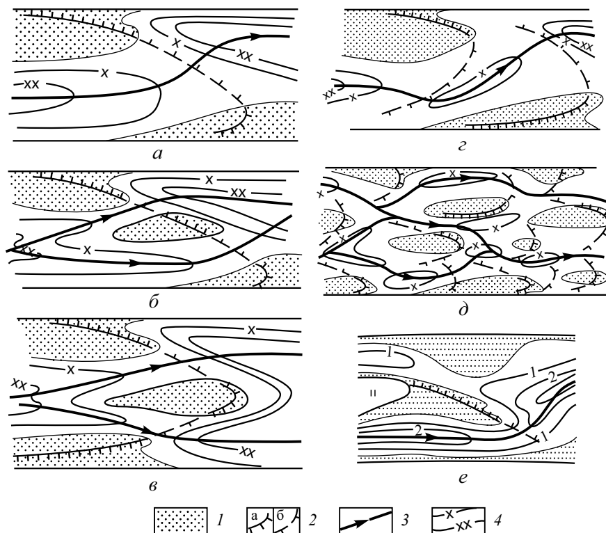
Рис. 4.45. Морфологические типы перекатов как грядовых форм руслового рельефа: a — перекат-перекосная гряда; б — то же с осередком; в — перекат-гряда с осередком и побочными, расположенными напротив друг друга у противоположных берегов; г — перекаты, образованные побочными-грядами; д — перекаты-россыпи; e — перекаты-косы; 1 — обсыхающие в межень отмели; 2 — подвалье гряд-макроформ ( a — на обсыхающих отмелях; б — подводные части); 3 — динамическая ось потока; 4 — изобаты
