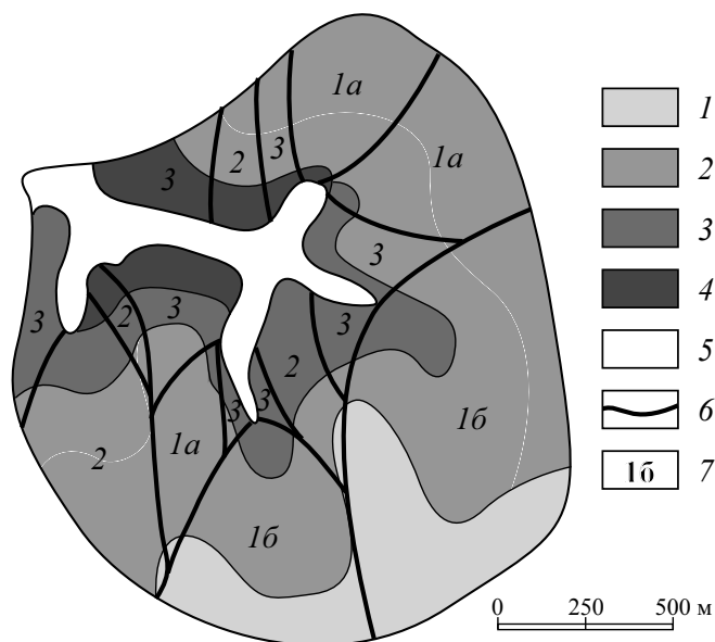
Рис. 6.2. Карта смыва почв со склонов водосбора балки Лапка и разделения склоновых водосборов на типы (1а, б, 2, 3 — см. табл. 6.2) по величине смыва почвы, т/га в год: 1–0–1; 2–1–2,5; 3–2,5–7,5; 4–7,5–10; 5 — днище балки; 6 — местные водоразделы; 7 — типы водосборов
