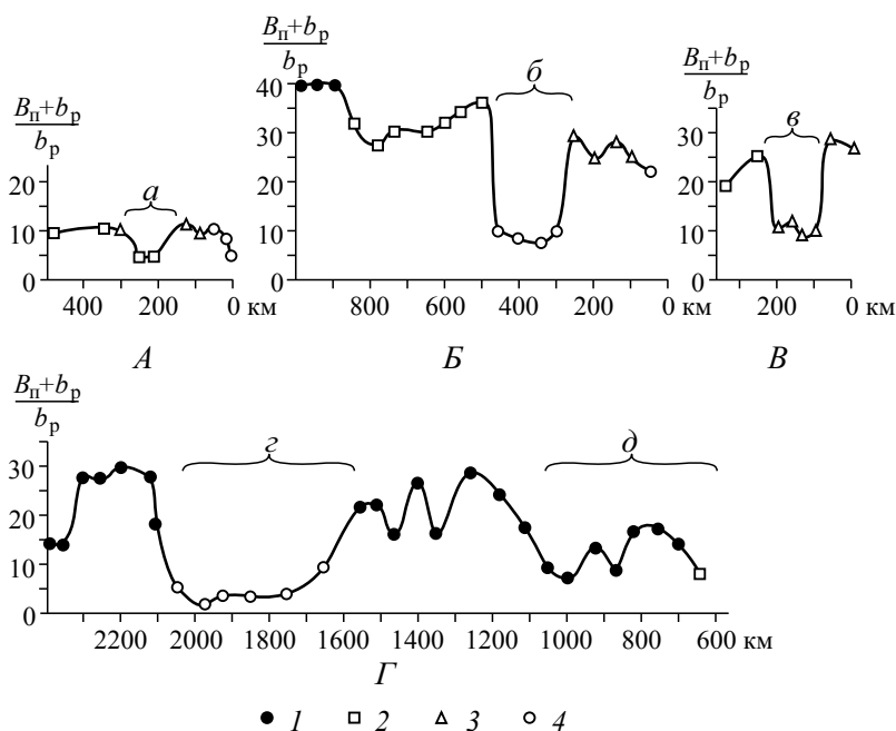
Рис. 4.68. Изменение относительной ширины поймы \frac{B_n + b_p}{b_p} , где B_n и b_p — соответственно ширина поймы и русла, по длине рек: А — р. Вилюй; Б — р. Таз; В — р. Омолуй; Г — р. Иртыш. Тектонические положительные структуры: а — Темирдяхское поднятие; б — Худосей-Большехетское поднятие; в — Сиэтиндэнское поднятие (хребет); з — Прииртышское поднятие; д — Вагайская антеклиза. Поймы: 1 — сегментно-гривистая; 2 — сегментно-гривистая; 3 — сегментно-островная и гривисто-островная; 4 — ложбинно-островная
