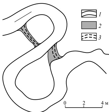
Рис. 4.51. Спряmlения излучины по бобровому ходу (Подмосковье): 1 — русло; 2 — новый участок русла; 3 — бобровые ходы
