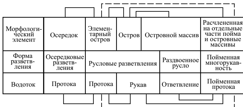
Рис. 4.34. Схема структуры разветвлений — осередковой, русловой (островной), пойменной и пути их эволюции (показаны стрелками) (по Р.С. Чалову и др. [2011], с изменениями)
