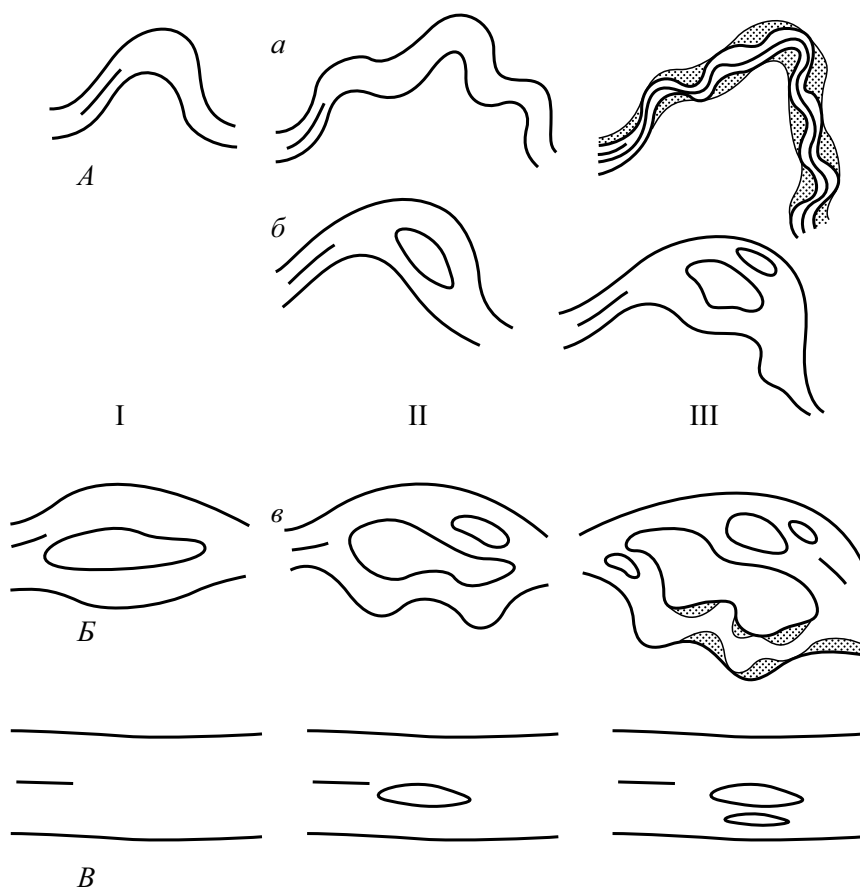
Рис. 4.27. Иерархия форм русла на излучинах (А), в разветвленном (Б), в прямолинейном русле (В); а, б, в-разновидности сочетаний русловых форм разных порядков. I — формы русла, определяющие его морфодинамический тип; II и III — формы русла, осложненные образованиями II и III порядков
