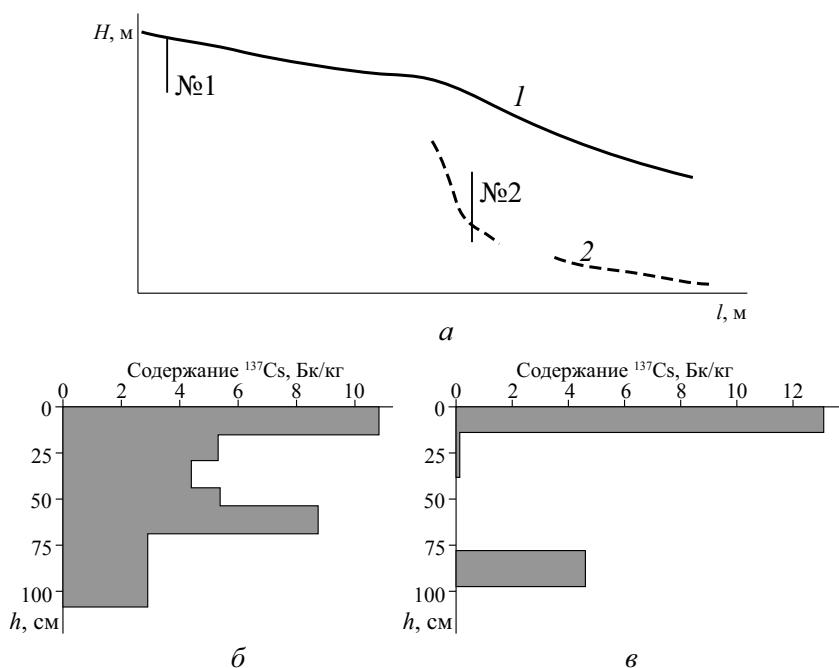
Рис. 3.17. Продольный профиль верховьев оврага Безымянный (Оренбургская область) и эпюры распределения Cs-137 в разрезах, расположенных до (разрез № 1) и ниже (разрез № 2) погребенной вершины оврага:
