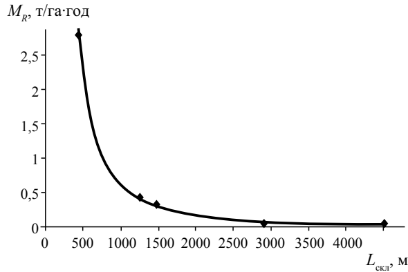
Рис. 2.27. Зависимость модуля стока наносов M_R от длины склона L_{скл} в одиночном ручье в диапазоне уклонов 1–6°
