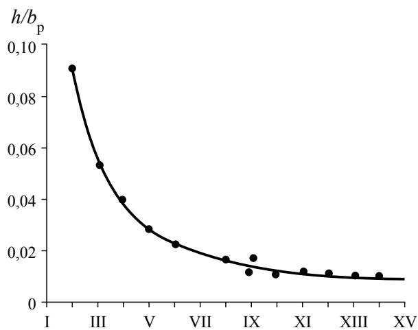
Рис. 4.22. Изменение относительной глубины русла h/b_p с увеличением порядка реки N_p [Ржаницын, 1985]
