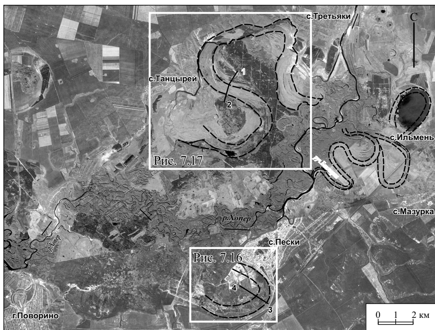
Рис. 7.15. Палеорула в долине р. Хопер между с. Третьяки и г. Поворино. Отмечены линии буровых профилей, показанных на рис. 7.16 и 7.17
