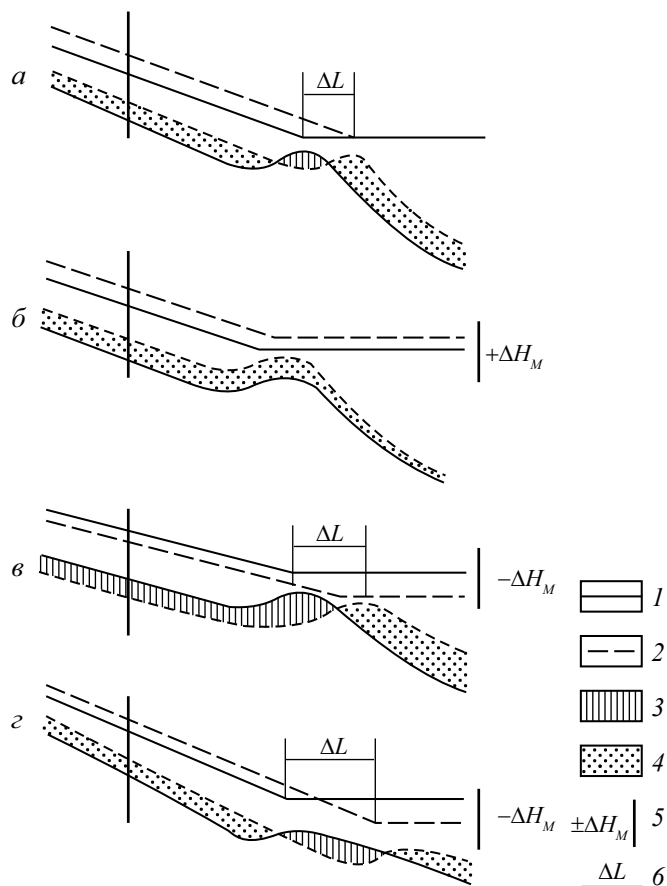
Рис. 5.8. Схема направленных русловых деформаций на устьевом участке реки (по В.Н. Михайлову [1997]):
