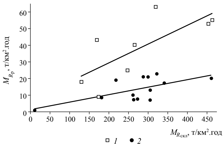
Рис. 6.8. Зависимость между модулями стока наносов реки M_{Rp} и стока наносов со склона M_{R_{\text{скл}}} для рек бассейна Оки: 1 — лесная зона и север лесостепи; 2 — лесостепь
