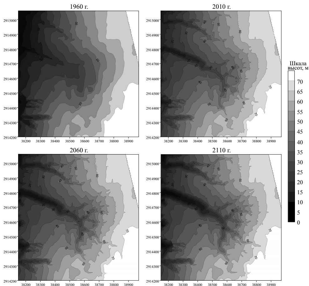
Рис. 3.6. Рассчитанная по динамической модели эволюция оврага Мботма-новый, проходившая в 2010–2110 гг. в условиях климата и землепользования конца XX в.
