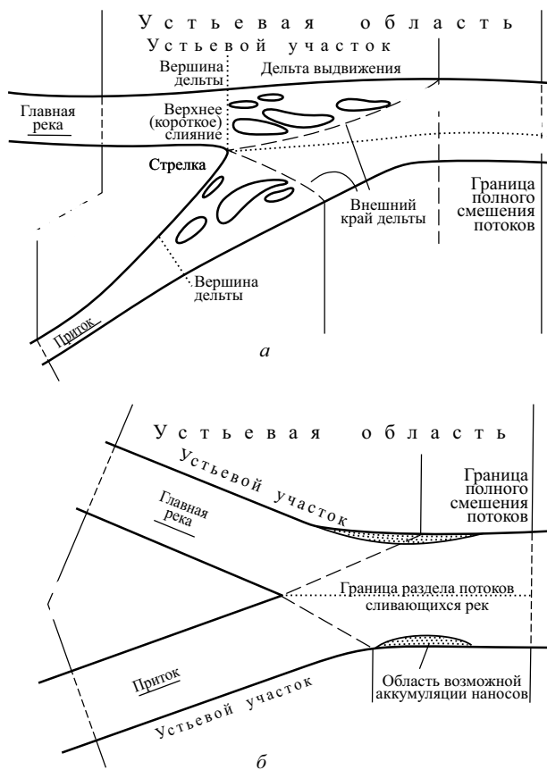
Рис. 4.43. Типы узлов слияния рек и их районирование: a — дельтовое; б — бездельтовое
