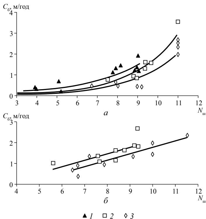
Рис. 4.49. Зависимость скорости размыва берегов C_6 от порядка реки N и уклона I : а — при отступлении берега вследствие размыва; б — вследствие размыва берега и оползневых процессов: 1 — при I = 0,2-0,3‰ ; 2 — при I = 0,1-0,2‰ ; 3 — при I < 0,1‰
