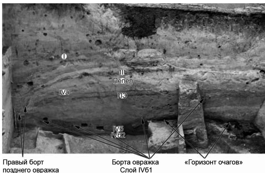
Рис. 7.2. Валдайский делювий и формы склоновой эрозии в археологическом раскопе К-14, 2-я терраса балки Покровский Лог, с. Костенки Воронежской области [Величко и др., 2009]
