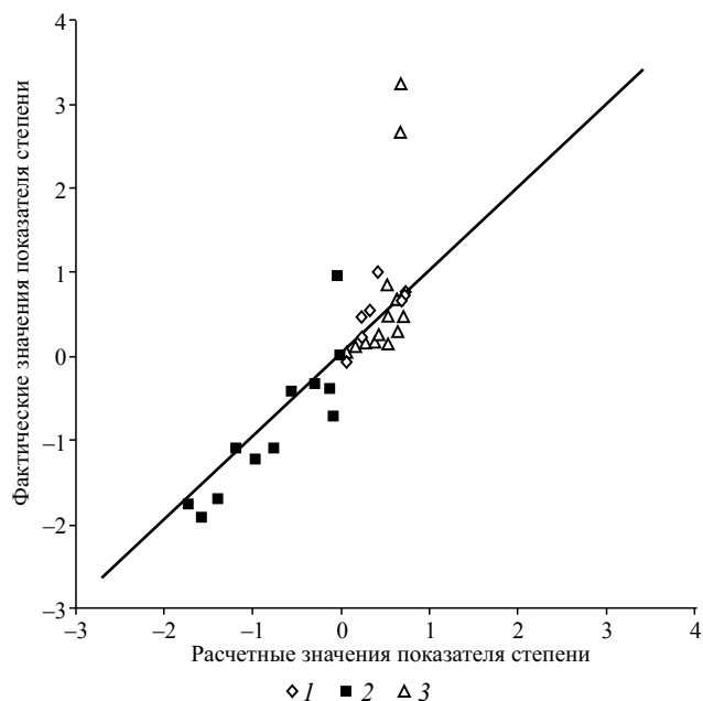
Рис. 2.14. Сопоставление расчетных и фактических значений показателя степени p при длине склона L_{\text{скл}} (по данным: 1 — Zhongshan, Xiuung, [1988]; 2 — Singh, Baby et al., [1981]; 3 — Нгуен Куанг Ми, [1995])
