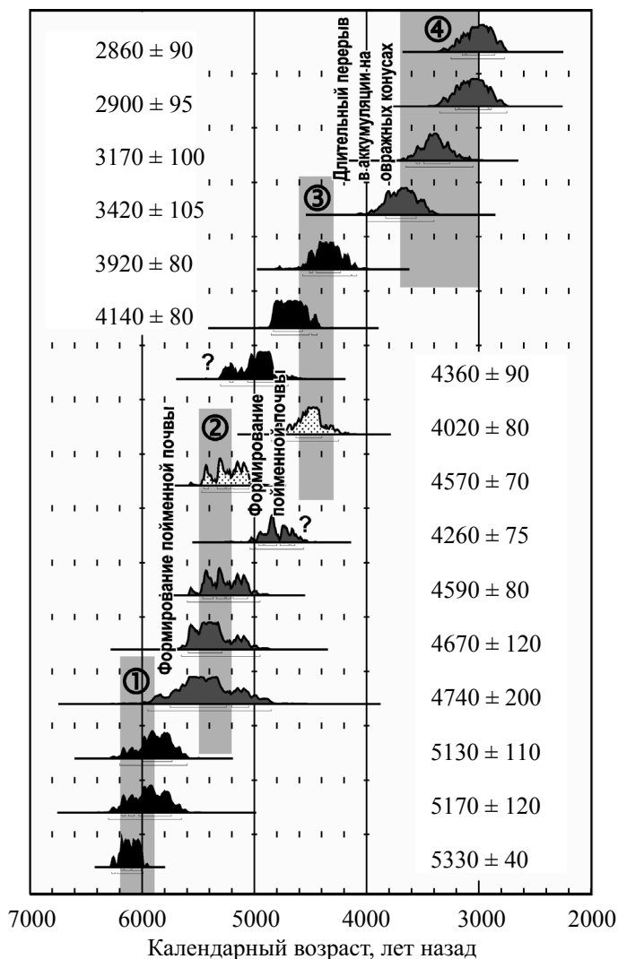
Рис. 7.8. Периоды высокой флювиальной активности (овражная эрозия, мощные паводки на реках) в бассейне р. Протвы (территория Боровской УНС МГУ, Калужская область) по данным ^{14}\text{C} датирования следов экстремальных палеогидрологических событий [Panin et al., 2011]. Интервалы высокой флювиальной активности (высокого стока) обозначены номерами в кружочках и показаны пунктирными полосами. Заливка серым графиков распределения вероятности ^{14}\text{C} дат обозначает их принадлежность к разным интервалам высокого стока; крапом — принадлежность к периодам низкого стока
