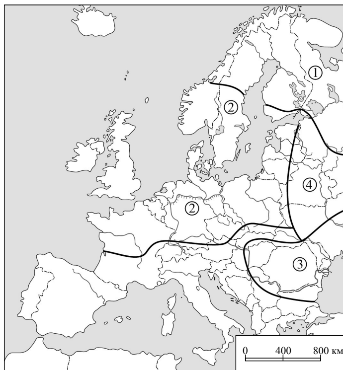
Рис. 2.22. Схема районирования равнин умеренного пояса Европы по преобладающему климатическому типу эрозии почв:
