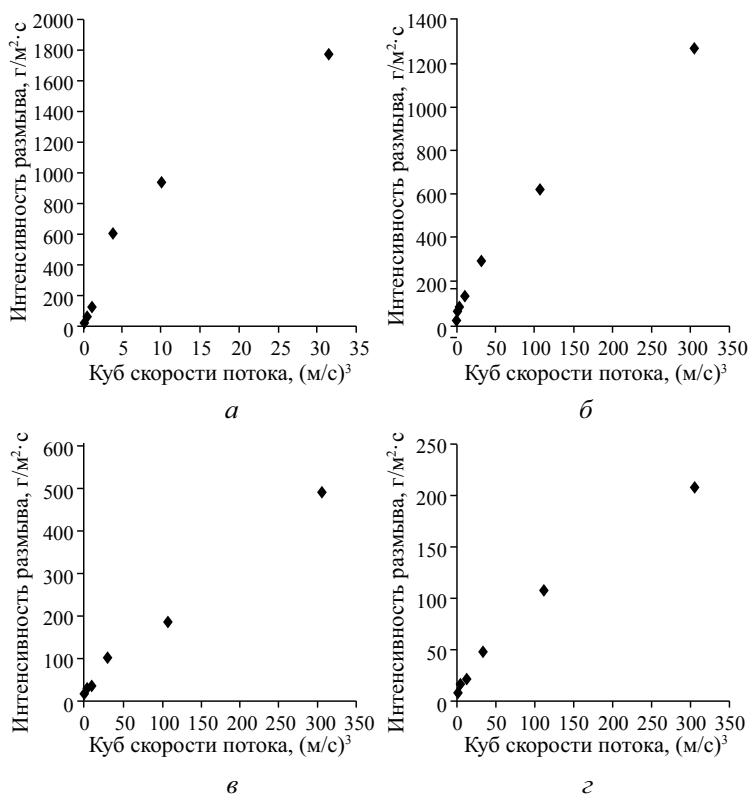
Рис. 2.11. Зависимость интенсивности размыва модельных образцов почвы различной плотности (а — 1,2 \text{ г/см}^3 ; б — 1,3 \text{ г/см}^3 ; в — 1,4 \text{ г/см}^3 ; г — 1,5 \text{ г/см}^3 ) от куба скорости V^3 в широком диапазоне скоростей (от 0,6 до 6,7 м/с)
