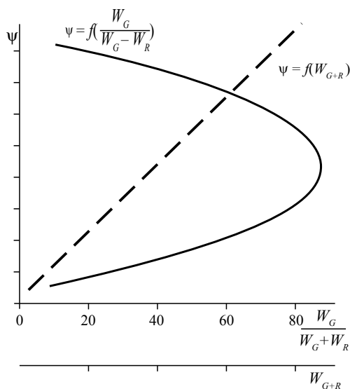
Рис. 4.60. Связь интегрального показателя морфологии русла и интенсивности его переформирования \psi от величины суммарного стока наносов W_{R+G} и доли стока влекомых наносов в нем
