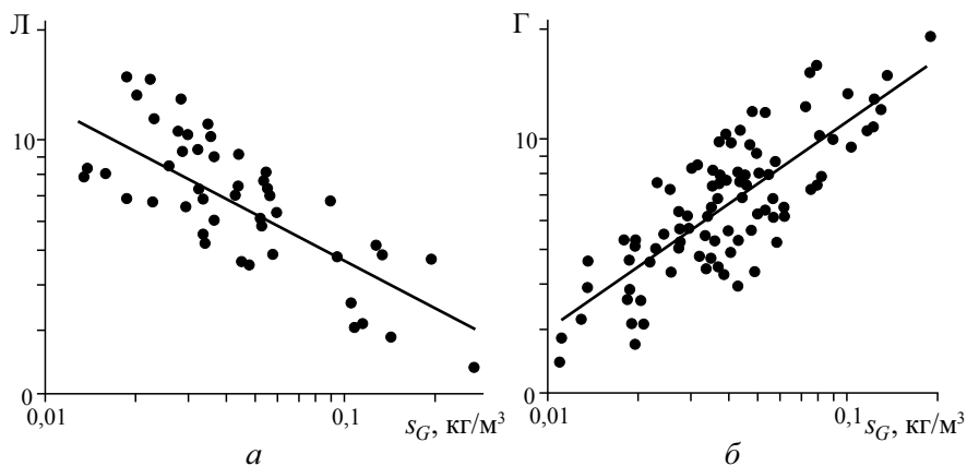
Рис. 4.63. Зависимость числа Лохтина L (а) и морфометрического параметра Глушкова \Gamma (б) от удельной величины стока влекомых наносов s_G [Резников, 2006]
