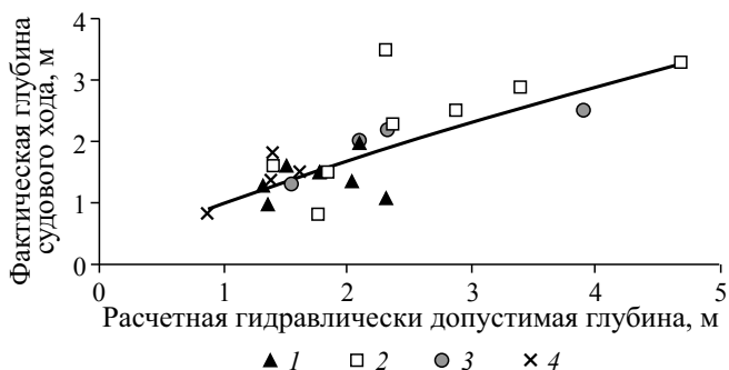
Рис. 8.15. Сопоставление гидравлически допустимых и фактических судоходных глубин для рек с разными типами русла и разными нарушениями русловых процессов: 1 — реки со слабоустойчивым песчаным руслом, меандрирующие или разветвленные; 2 — реки в нижних бьефах гидроузлов; 3 — реки с русловыми карьерами; 4 — реки с гравийно-галечными руслами
